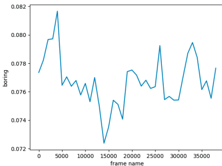
Рис. 5. Значения MSE по диапазонам фреймов для «Boring»
