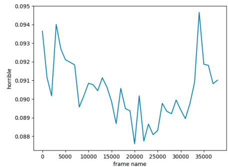
Рис. 8. Значения MSE по диапазонам фреймов для «Horrible»
