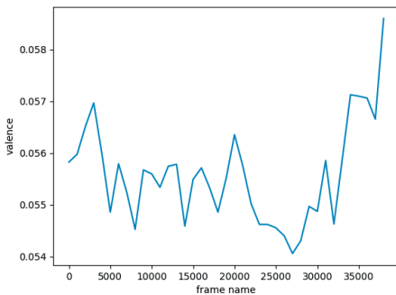
Рис. 4. Значения MSE по диапазонам фреймов для «Valence»
