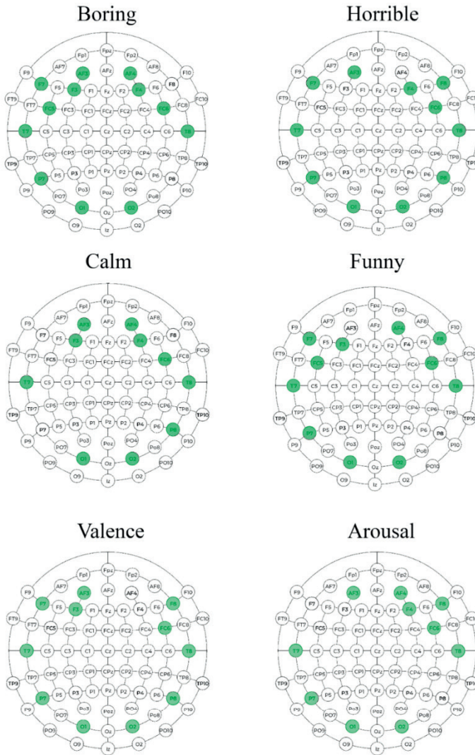
Рис. 2. Схемы расположения отобранных электродов
