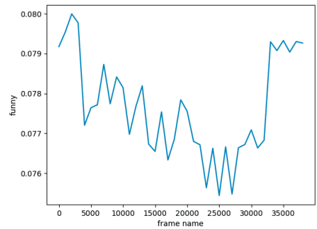
Рис. 7. Значения MSE по диапазонам фреймов для «Funny»
